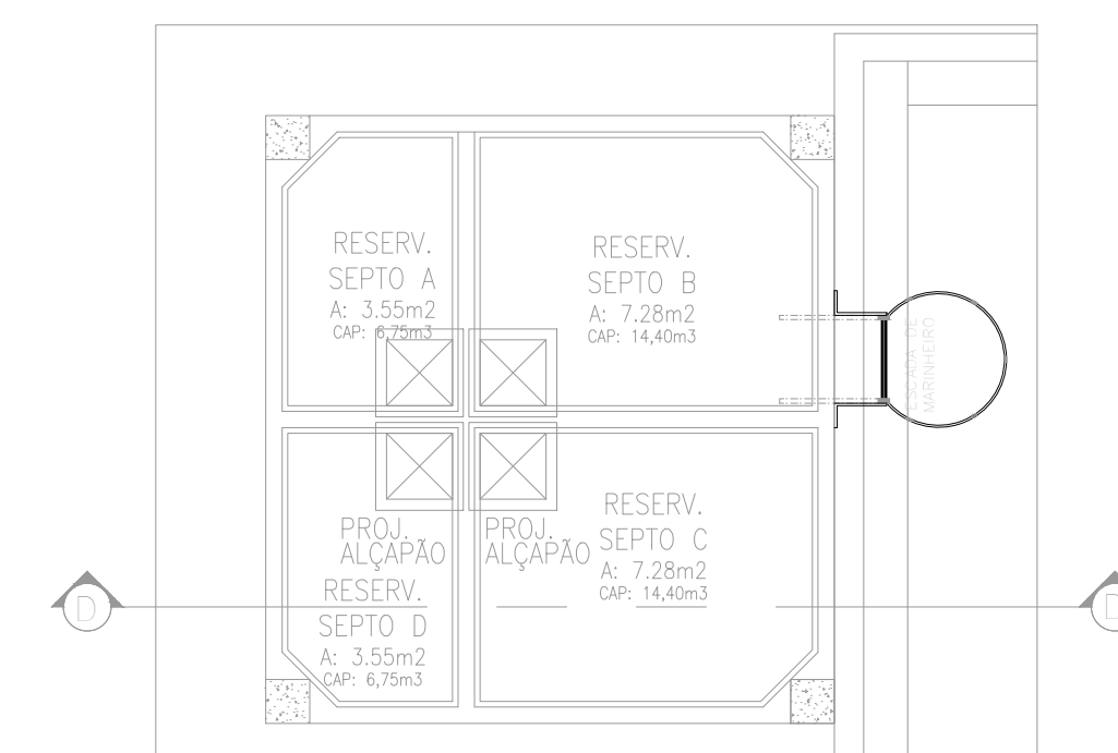
PLANTA BAIXA - RESERVATÓRIO ESCALA 1/75
