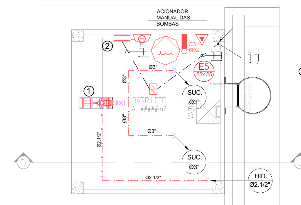
PLANTA BAIXA - BARRILETE ESCALA 1/75
