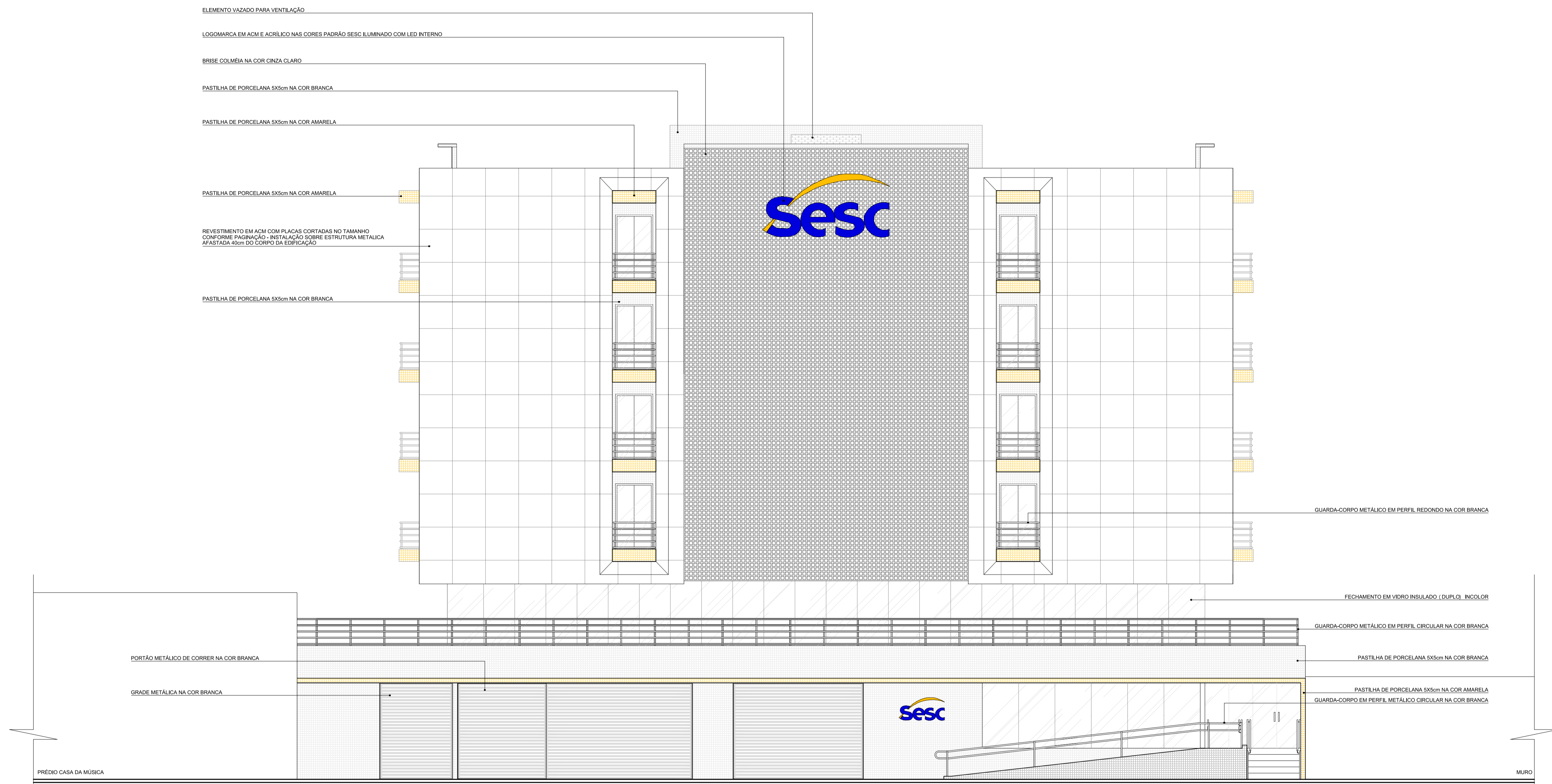
ELEVAÇÃO 01 ESC: 1/75
