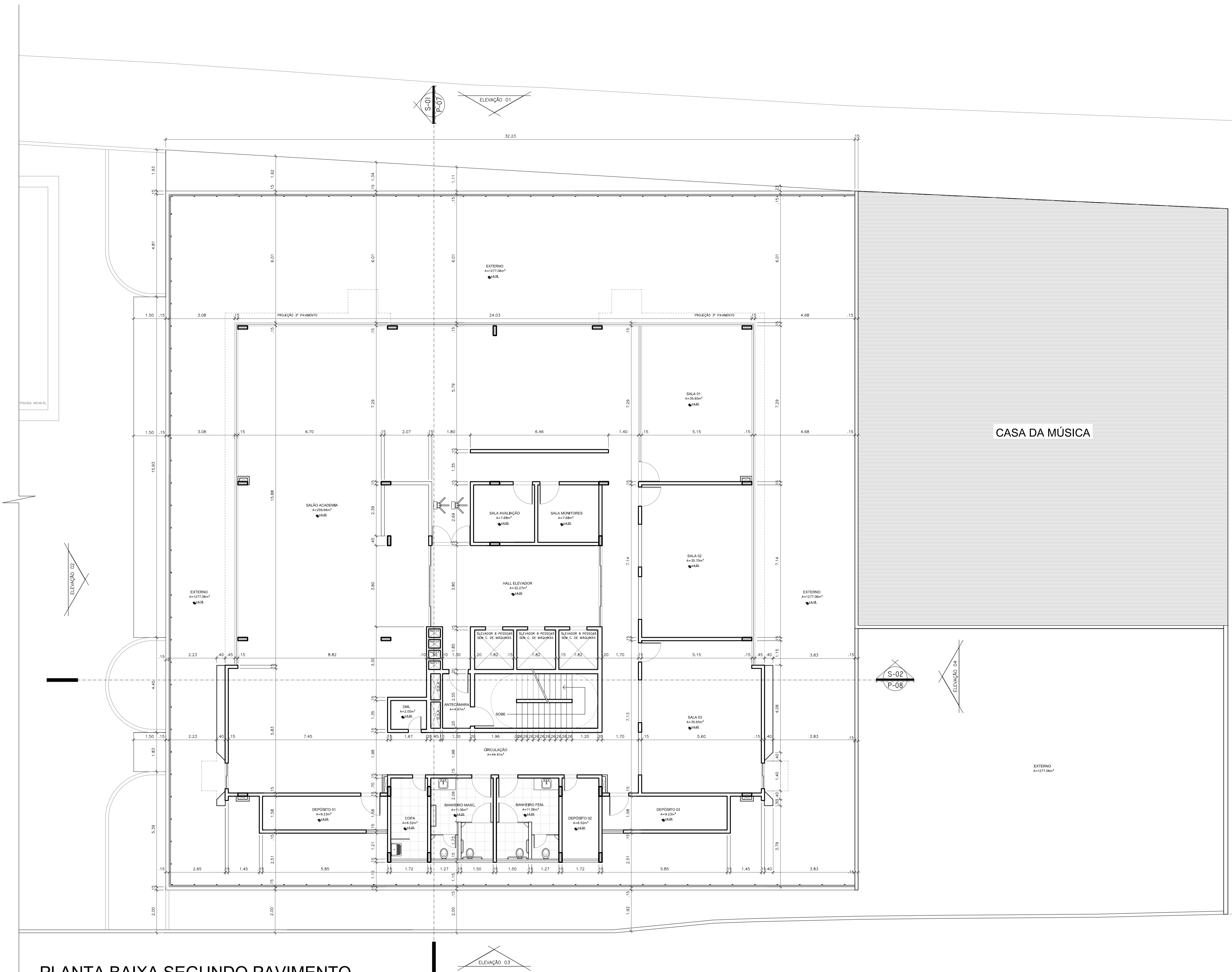
PLANTA BAIXA SEGUNDO PAVIMENTO ESC: 1/100
