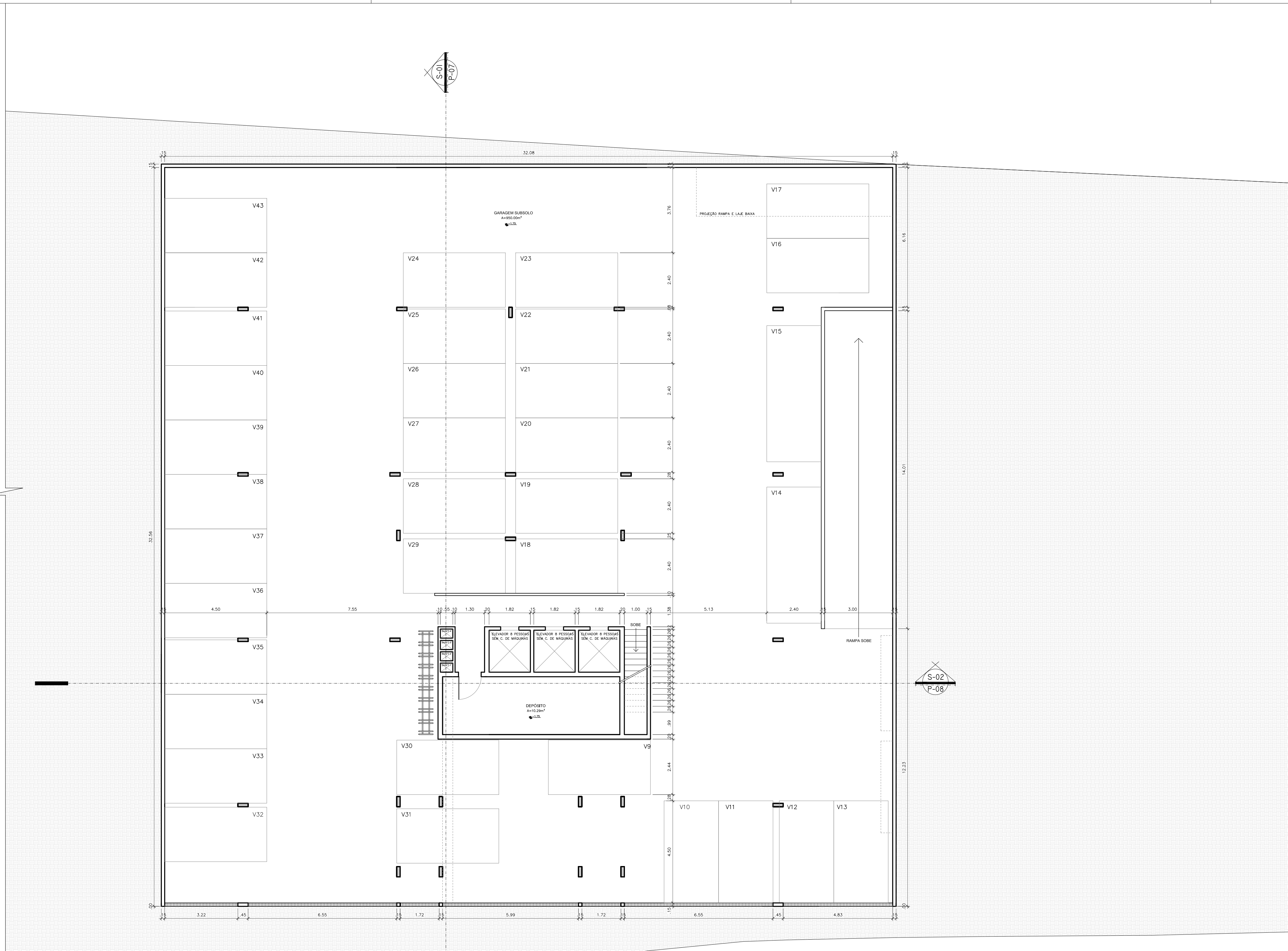
PLANTA BAIXA SUBSOLO ESC: 1/100
