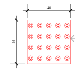
DETALHE 02 - MODULAÇÃO DO PISO Esc.: 1/10
