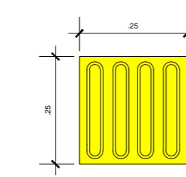
DETALHE 01 - MODULAÇÃO DO PISO Esc.: 1/10
